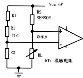
温度补偿电路
